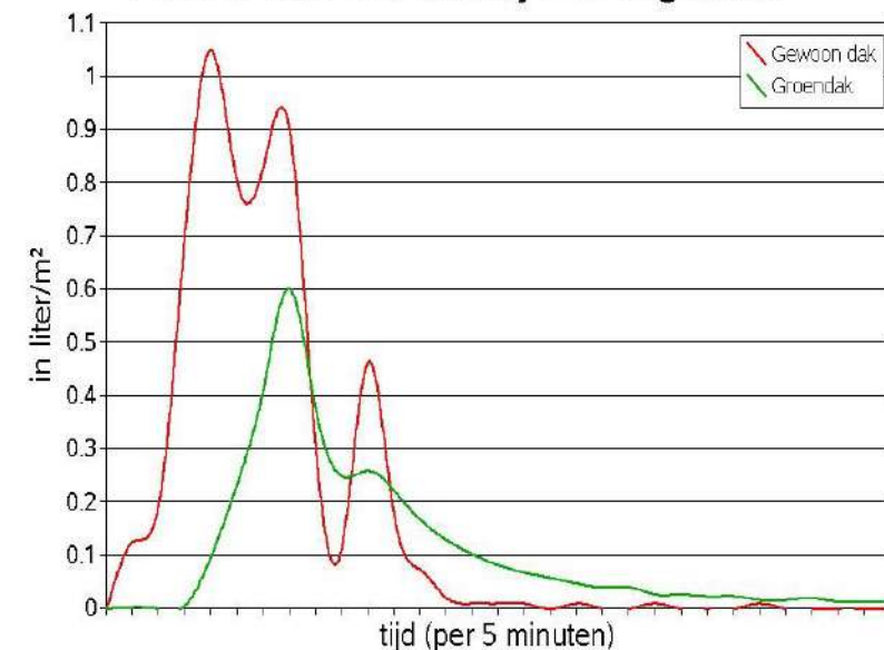
Afvoer van het dak bij een regenbui
