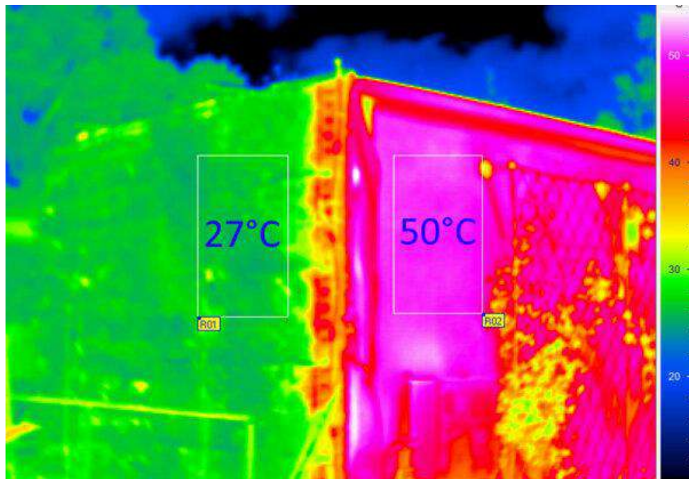
Muur met gevelgroen Muur zonder gevelgroen
